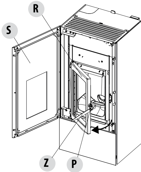
FIREBOX DOOR
